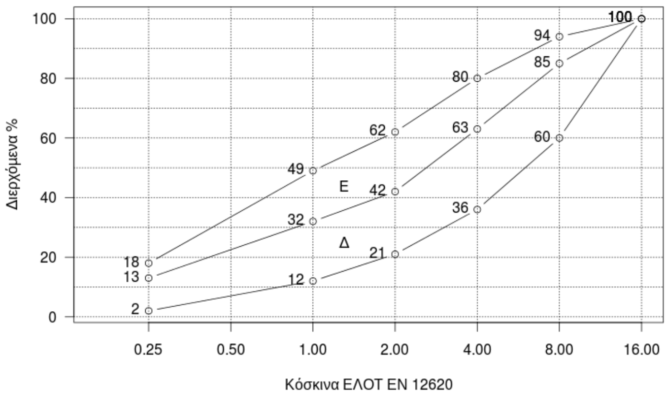
Διάγραμμα ΠΒ1 -3: Ορια κοκκομετρικής διαβάθμισης μίγματος αδρανών μέγιστου κόκκου 16mm.
