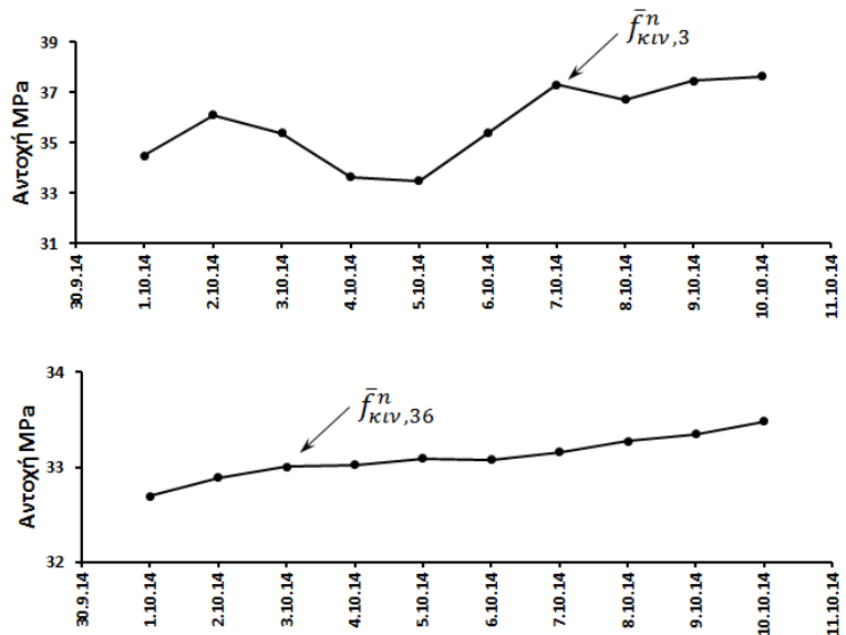
Σχ.: Β5-1 - Διάγραμμα της μεταβολής του \bar{f}_{κιν,3}^n και του \bar{f}_{κιν,36}^n
